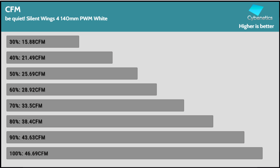
Fan Percentage Power
