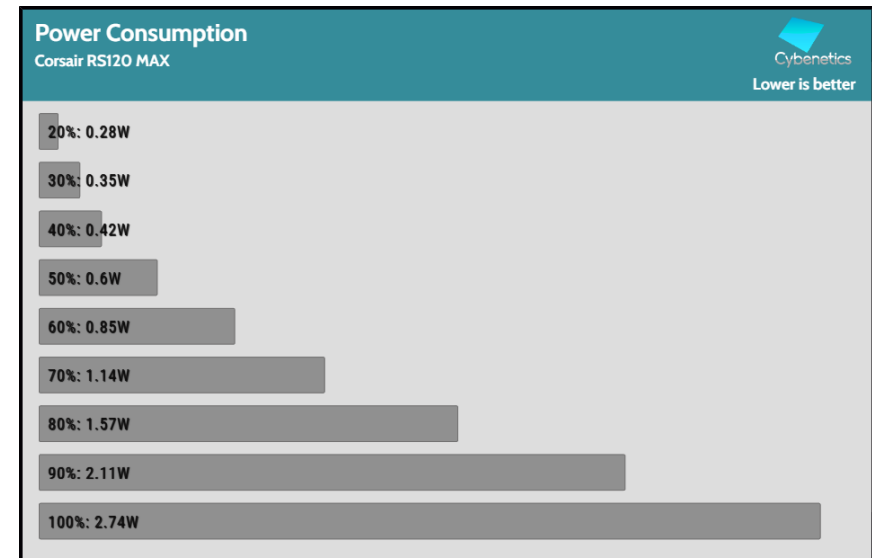
Fan Percentage Power
