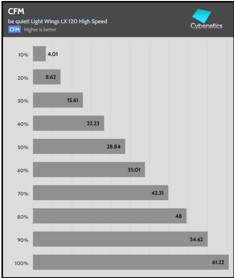
Fan Percentage Power
