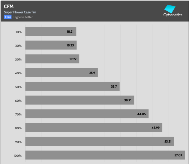
Fan Percentage Power
