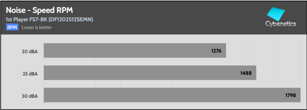
Fan Noise Speed
