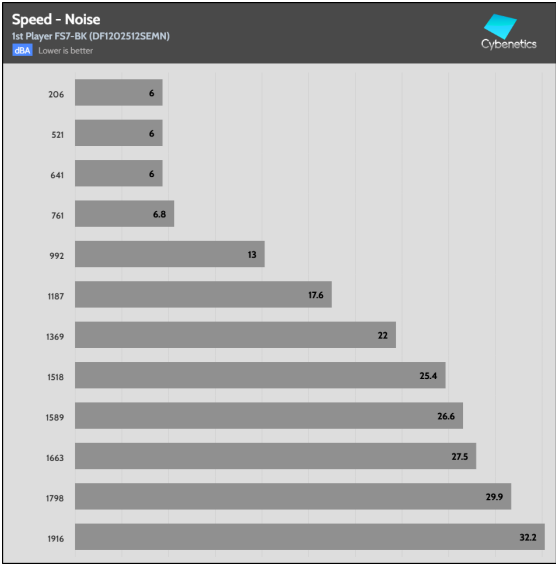
Fan Speed Noise
