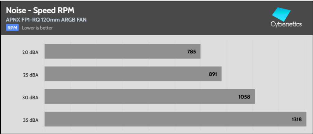
Fan Noise Speed
