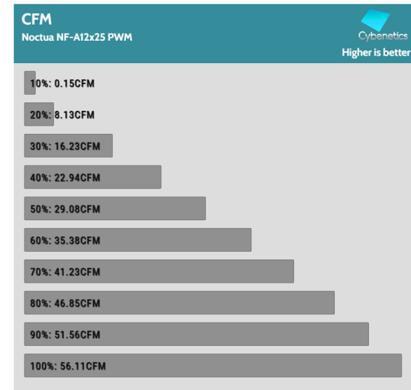
Fan Percentage Power
