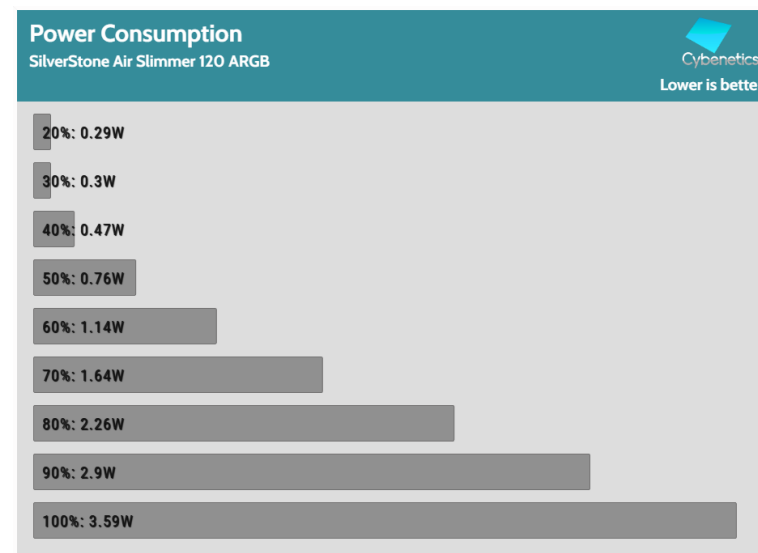
Fan Percentage Power
