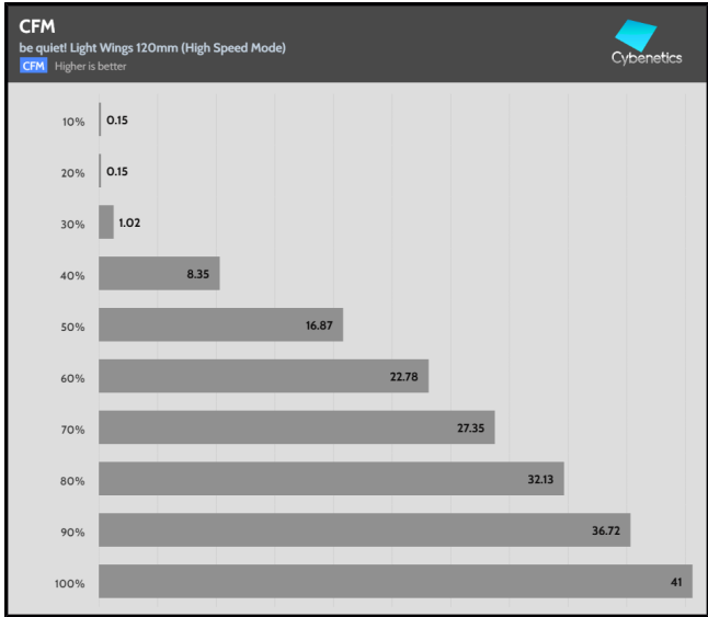
Fan Percentage Power
