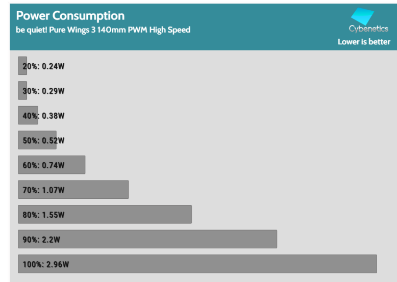
Fan Percentage Power
