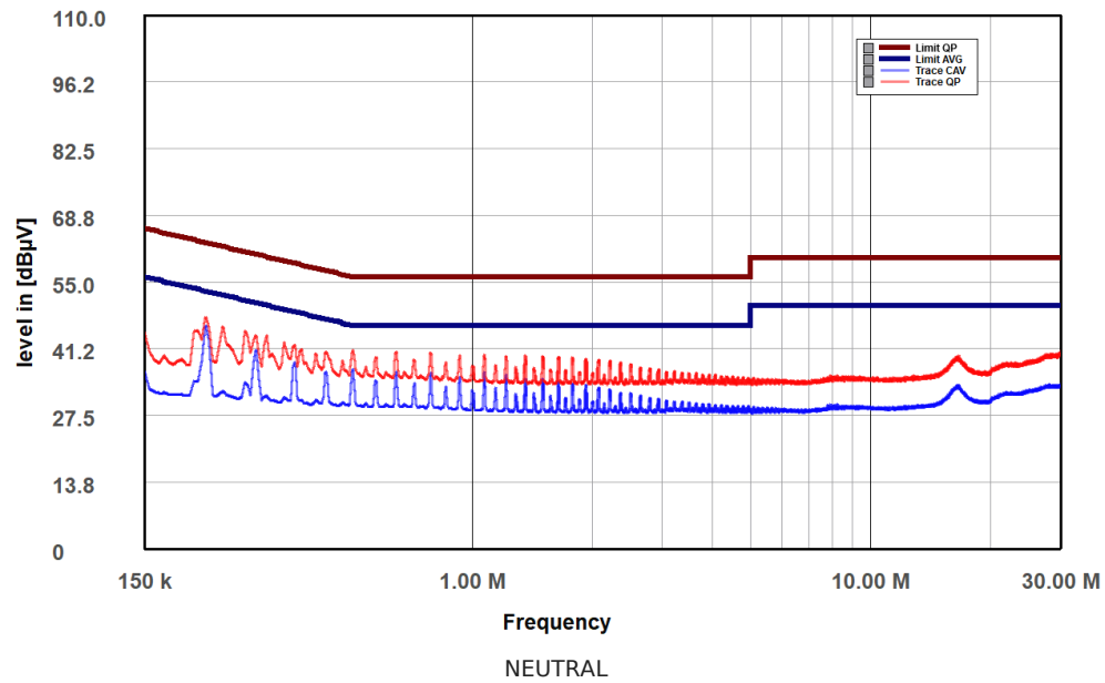
Lian Li SX0850P (LL85003049) Neutral
