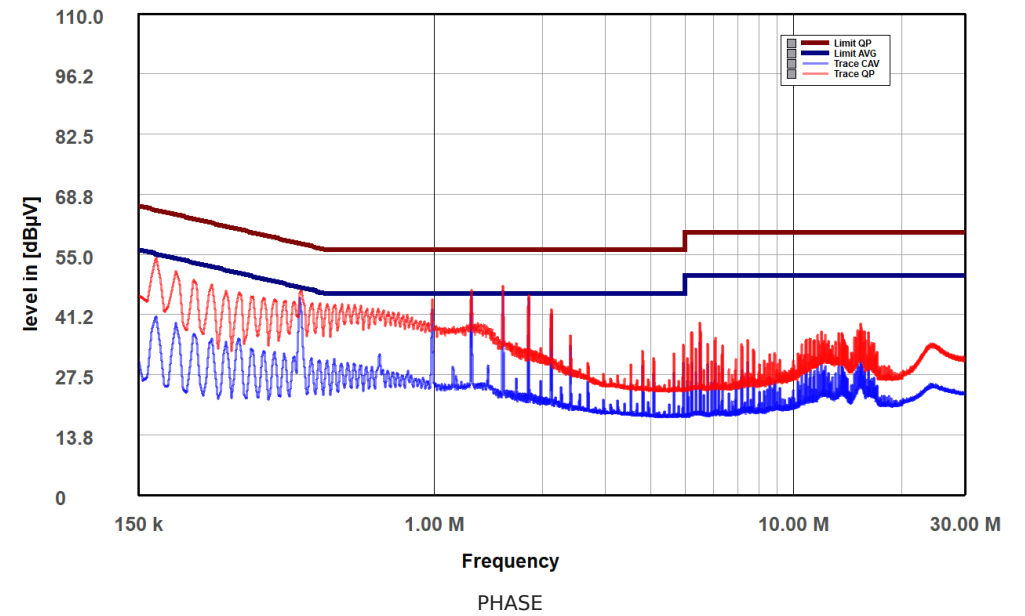
Gigabyte UD 1300W (GB13003306) Phase
