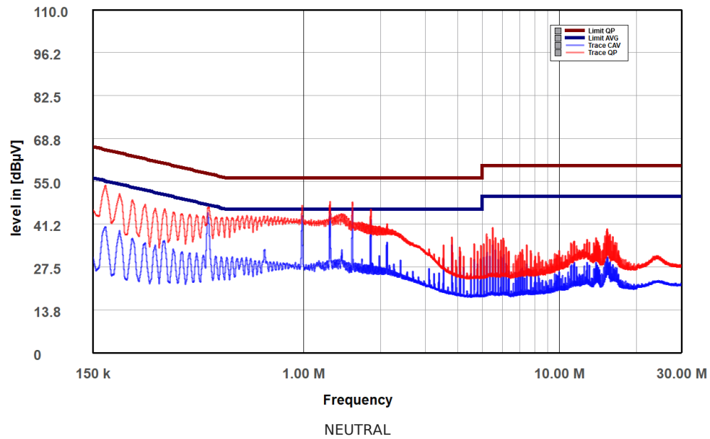
Gigabyte UD 1300W (GB13003306) Neutral
